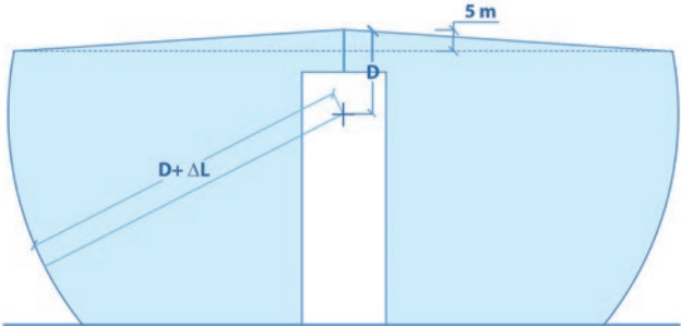
Fig 4 – Volumen protegido con pararrayos PDC.
