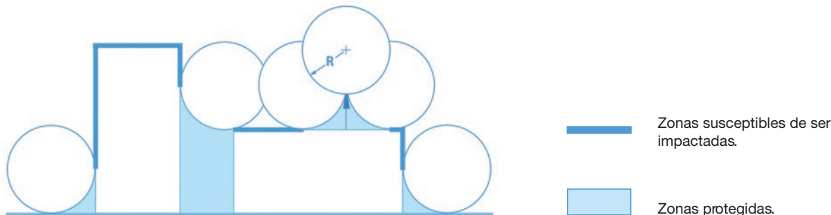
Fig. 3 – Esfera rodante en estructuras
